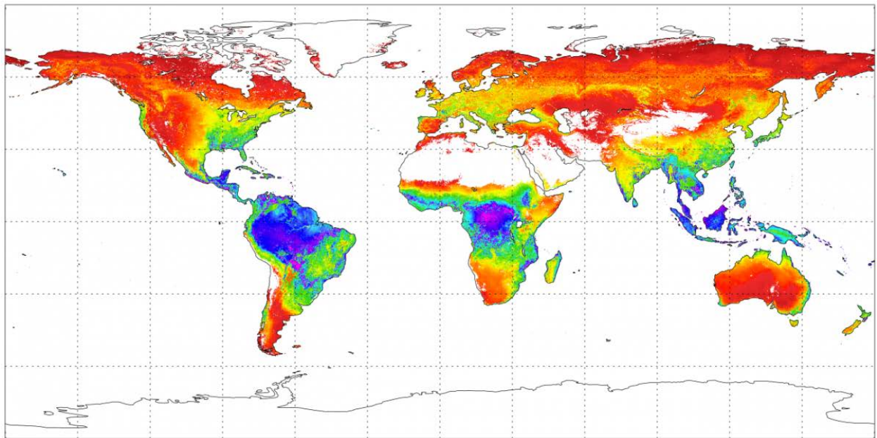
0 250 500 750 1000 1250 1500 Global Annual MOD16 ET (2000-2006) mm/yr
